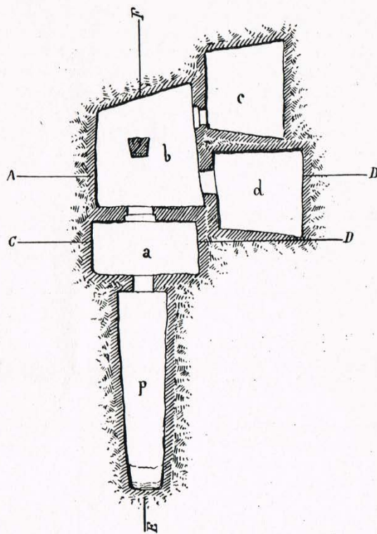
FIG. 34. - Pianta della tomba XIX. Scala 1:100.
