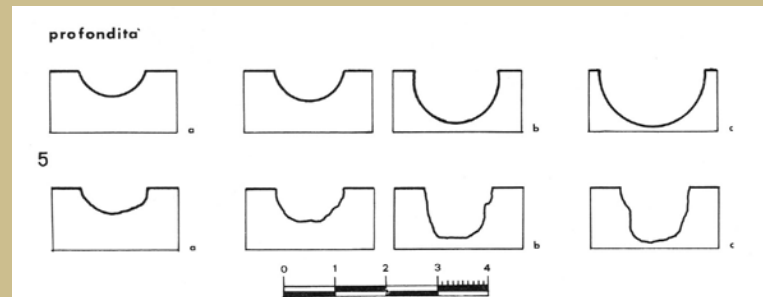
Fig. 3. Tipologie di sezione del solco e dei margini, larghezza e profondità (cfr. pp. 18-19).
